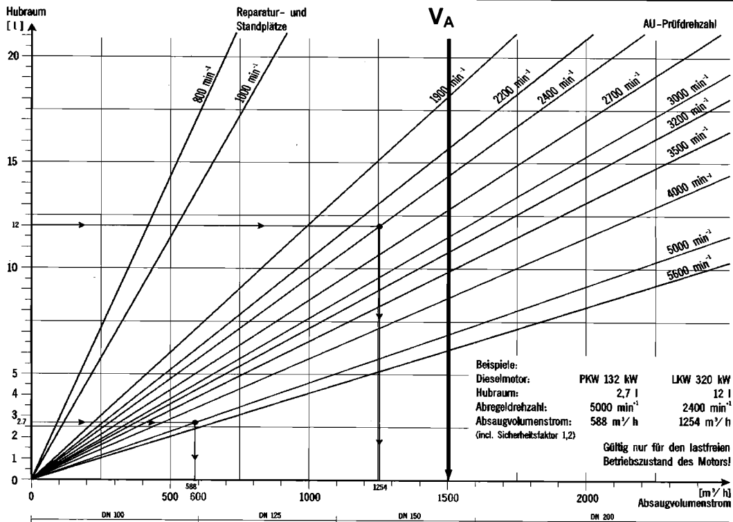
Diagramm zur Bestimmung des Absaugvolumenstromes im Bereich von Reparatur- und AU-Prüfplätzen
